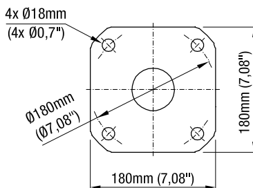
Размеры фланца емкости
